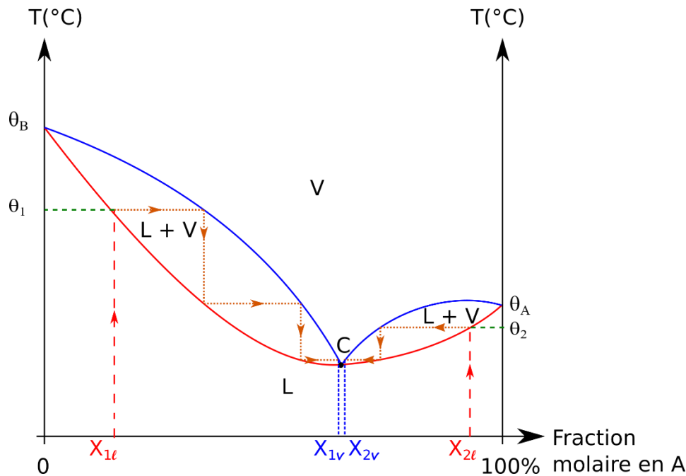
Figure 10 : Distillation fractionnée d'un mélange azéotropique
