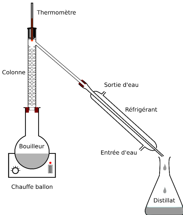
Figure 4 : Distillation fractionnée
