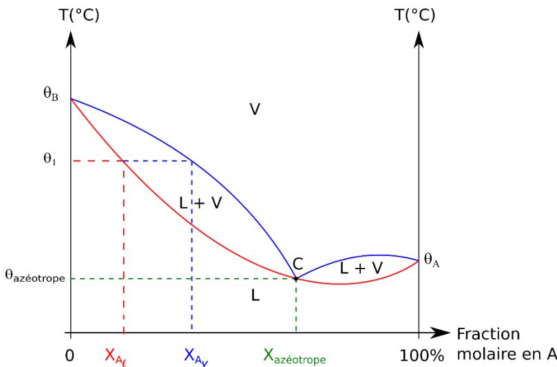
Figure 9 : diagramme binaire d'un mélange azéotropique
