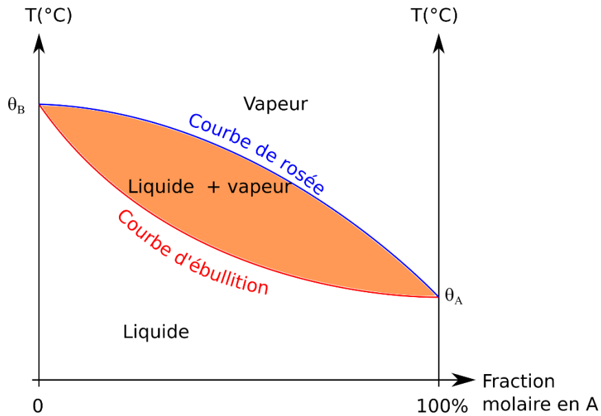
Figure 5 : diagramme isobare d'équilibre liquide-vapeur d'un mélange binaire
