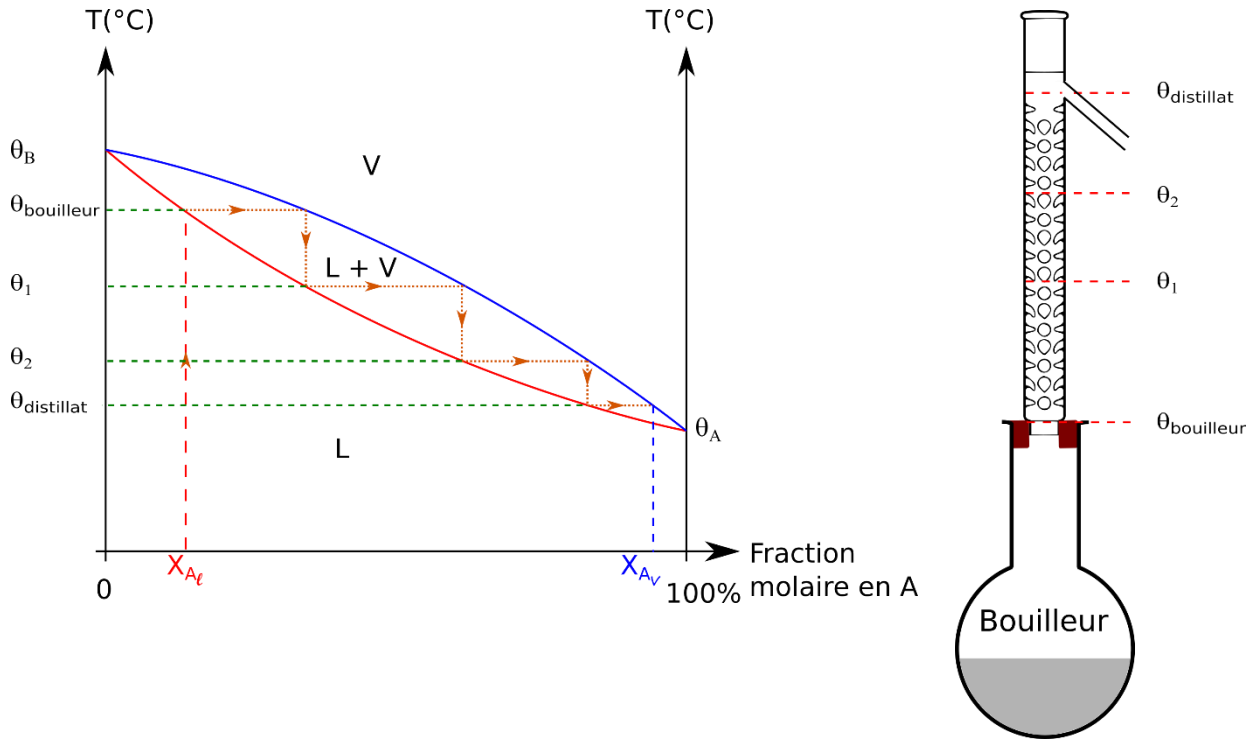
Figure 8 : distillation fractionnée
