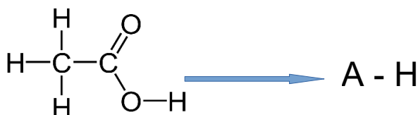
Figure 1: Acide éthanoïque : formule développée
